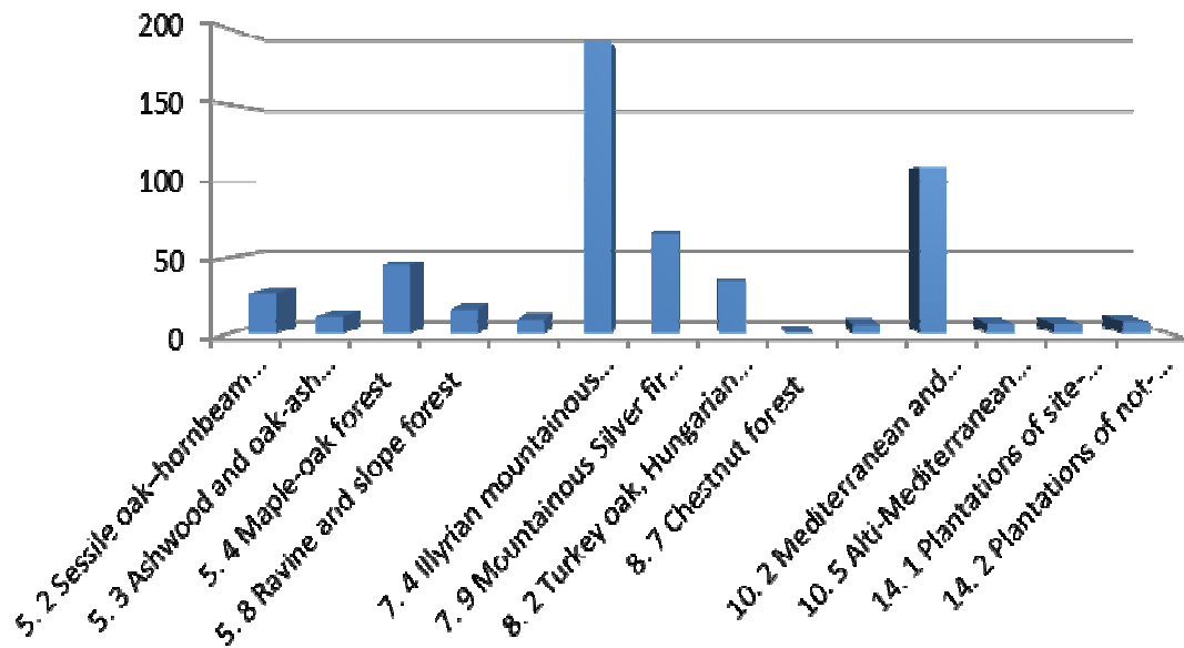
Fig.7. Productivity per forest type
