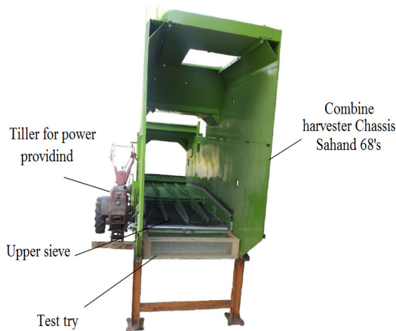
Fig 4. Test stand
